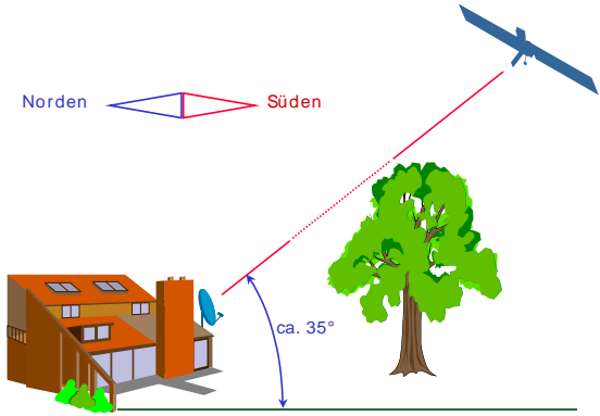
Freie Sicht nach Süden ist eine Grundvoraussetzung für guten Satellitenempfang
